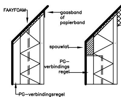
aansluiting schuin dak PG60 system
