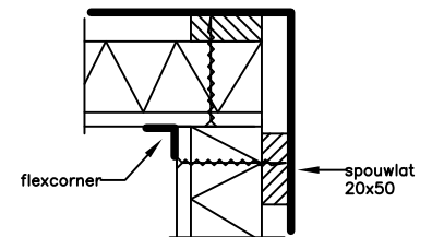
inwendige hoek PG60 system
