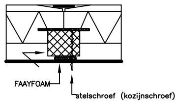
koppeling PG60 system op oneffen wand
