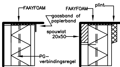
plafondaansluiting PG60 system
