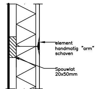
stuiknaad PG60 system, op toppen
