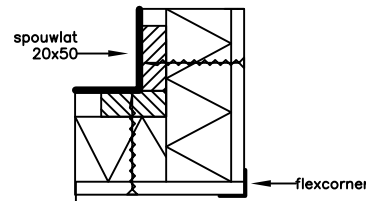
uitwendige hoek PG60 system
