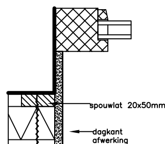
kozijnaansluiting PG60 system
